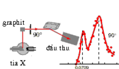
Hình 7-7. Thí nghiệm Compton
