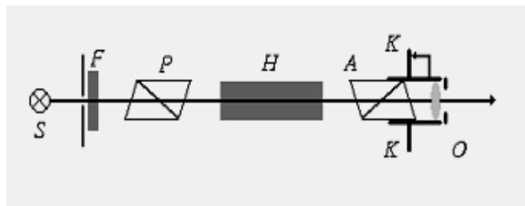
Hình 5-18. Mô hình của đường kế
