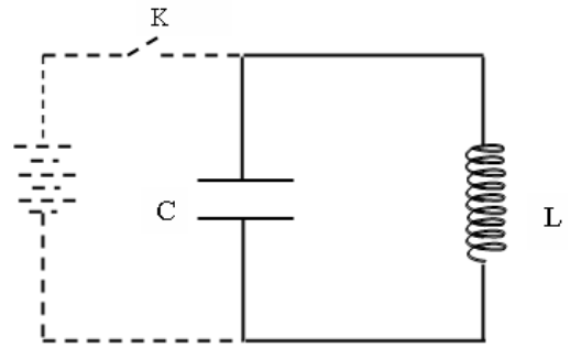
Hình 1-6. Mạch dao động điện từ riêng
