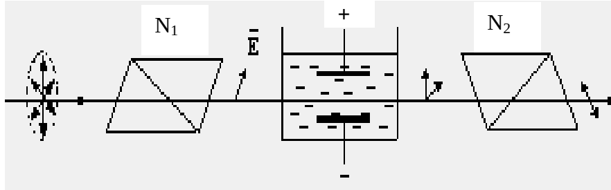
Hình 5-16. Thí nghiệm về hiệu ứng Kerr
