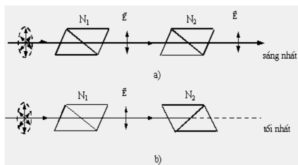
Hình 5-10. a) Hai nicol song song; b) Hai nicol bắt chéo
