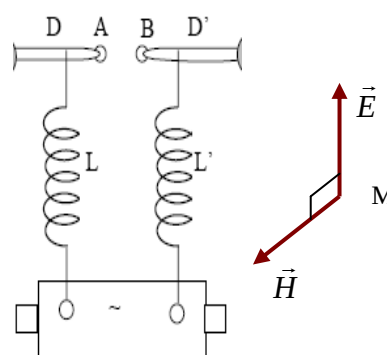
Hình 1-35. Thí nghiệm Hertz
