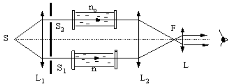
Hình 2-18. Giao thoa kế Rayleigh
