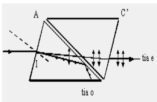
Hình 5-9. Lăng kính Nicol
