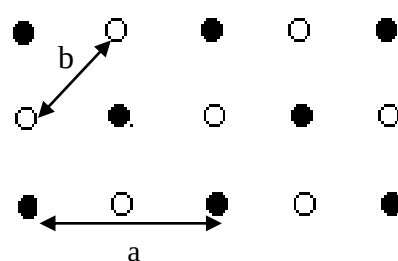
Hình 10-1. Mạng tinh thể hai chiều
