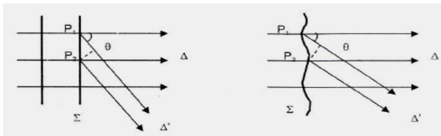
Hình 4-5. Sự tán xạ ánh sáng
