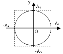
Hình 1-19. Quỹ đạo của chất điểm khi
