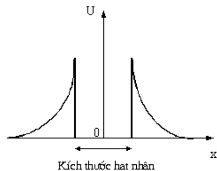
Hình 8-9. Hiện tượng phân rã \alpha
