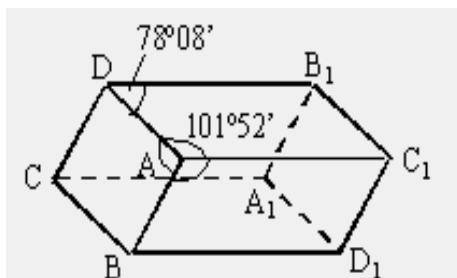
Hình 5-7. Tinh thể băng lan
