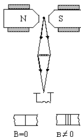
Hình 9-9. Hiệu ứng Zeeman
