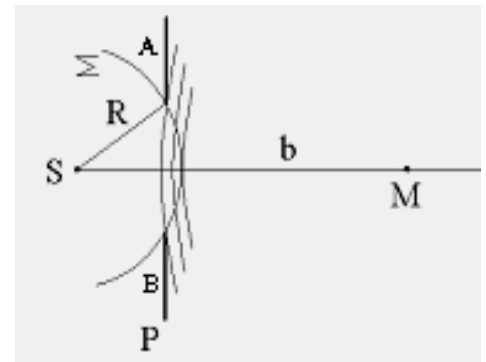
Hình 3-4. Nhiễu xạ qua lỗ tròn
