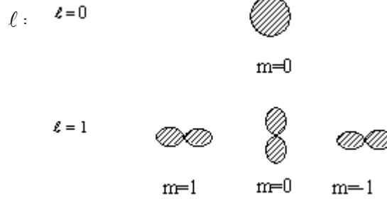
Hình 9-4. Phân bố electron theo góc đối với trạng thái s ( \ell=0 ) và p ( \ell=1 )
