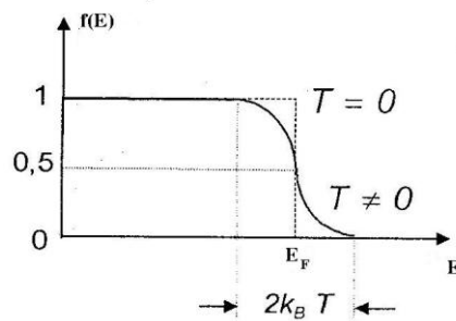
Hình 10-6. Hàm phân bố Fermi-Dirac
