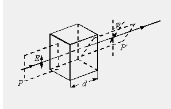
Hình 5-17: Hiện tượng quay mặt phẳng phân cực
