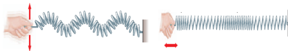
Hình1-22. Mô tả sóng ngang và sóng dọc
