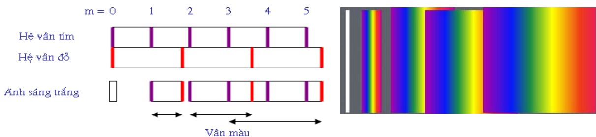
Hình 2-11. Giao thoa gây bởi ánh sáng trắng
