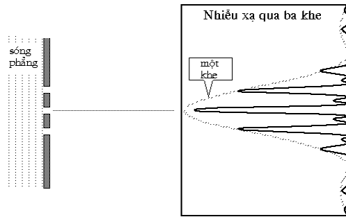
Hình 3-11. Ảnh nhiễu xạ qua ba khe hẹp
