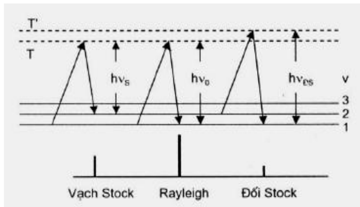
Hình 4-7. Sơ đồ mức năng lượng tán xạ Raman
