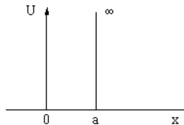
Hình 8-6. Giếng thế năng
