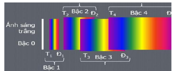
Hình: 3-13. Nhiễu xạ ánh sáng trắng
