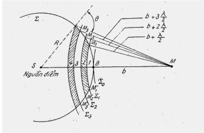
Hình 3-3. Đới cầu Fresnel
