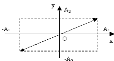
Hình 1-16. Quỹ đạo của chất điểm khi \varphi_2 - \varphi_1 = 2k\pi
