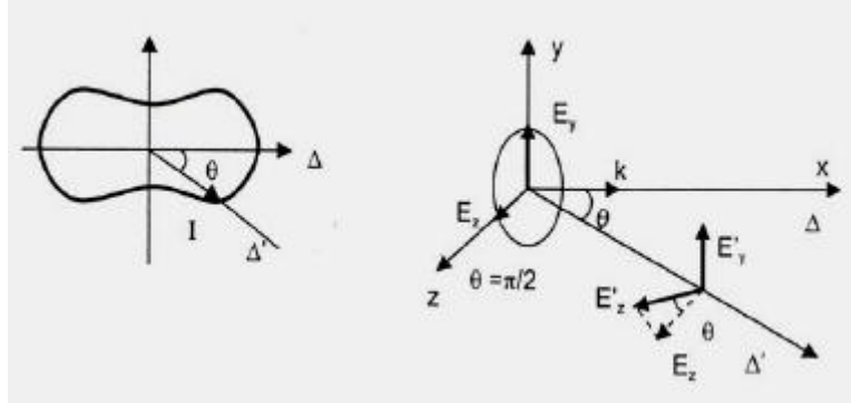
Hình 4-6. a. Phân bố cường độ ánh sáng tán xạ theo phương quan sát. b. Sự phân cực của ánh sáng tán xạ.
