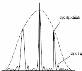
Hình 3-12. Phân bố cường độ giữa hai cực tiểu chính
