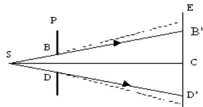
Hình 3-1. Hiện tượng nhiễu xạ ánh sáng
