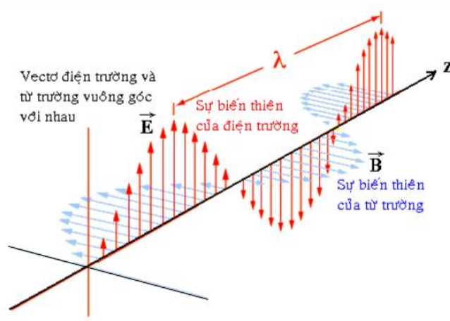
Hình 2.1. Ánh sáng lan truyền dưới dạng sóng
