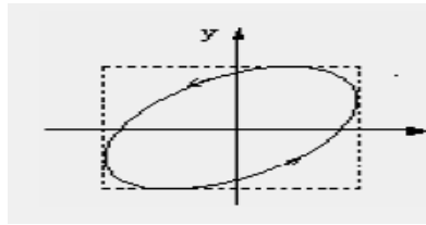
Hình 1-20. Các dạng quỹ đạo của chất điểm khi \varphi_2 - \varphi_1 = 0 \div 2\pi và A_1 = A_2
