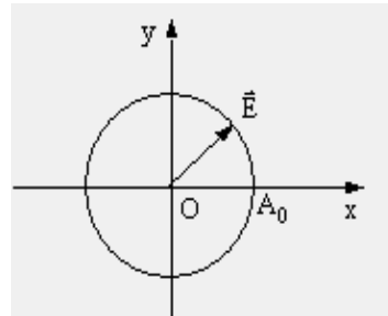
Hình 5-12b. Phân cực tròn
