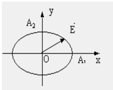
Hình 5-12a. Phân cực elip dạng chính tắc
