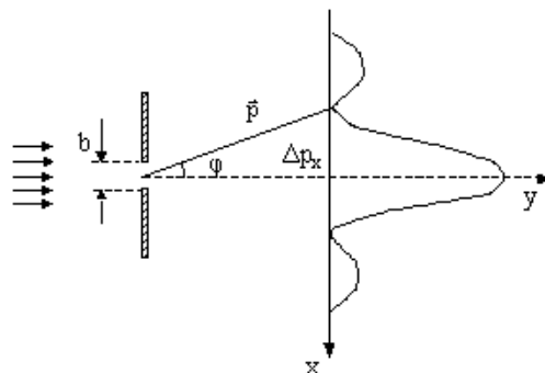
Hình 8-4. Nhiễu xạ electron qua khe hẹp
