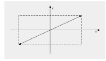
Hình 1-20. Các dạng quỹ đạo của chất điểm khi \varphi_2 - \varphi_1 = 0 \div 2\pi và A_1 = A_2
