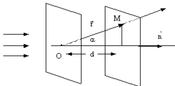
Hình 8-1. Sự truyền sóng phẳng ánh sáng
