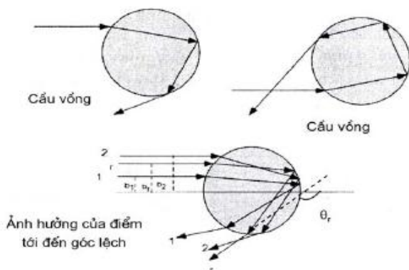
Hình 4-19. Sự lệch của tia nắng qua giọt mưa
