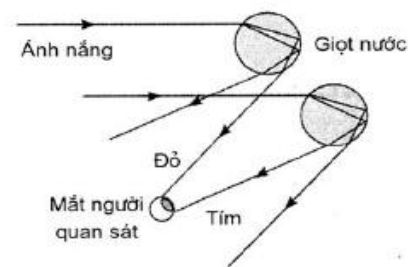
Hình 4-12. Đường đi của các tia sáng tới mắt từ các giọt mưa
