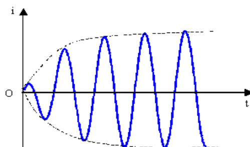
Hình 1-12. Đường biểu diễn
