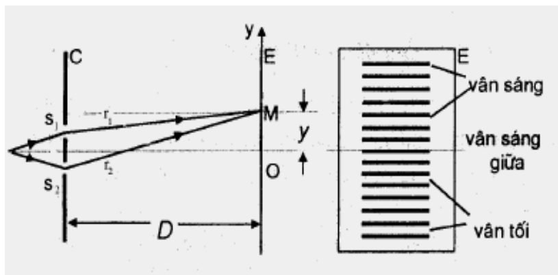
Hình 2-7. Sơ đồ thí nghiệm giao thoa với hai khe
