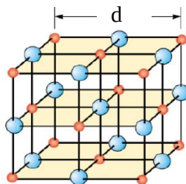
Hình 3-14. Sơ đồ biểu diễn mạng tinh thể
