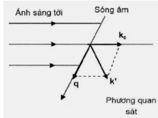
Hình 4-8. Tán xạ Mandelstam – Brillouin
