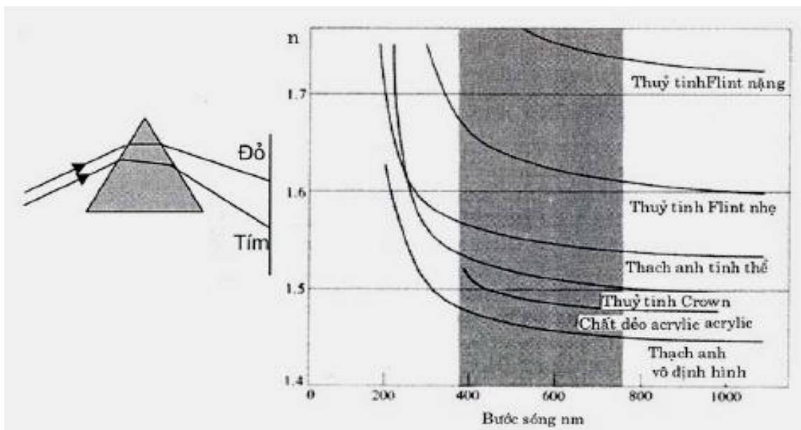
Hình 4-1. Sự tán sắc và đường cong tán sắc
