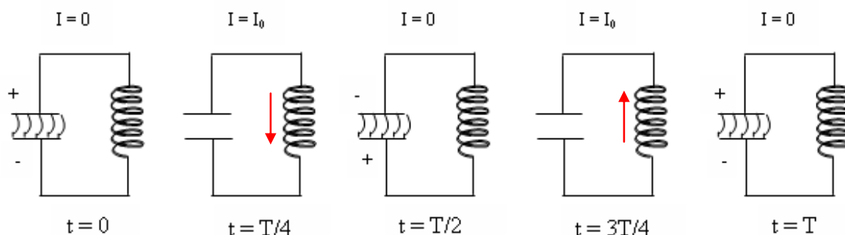
Hình 1-7. Quá trình tạo thành dao động điện từ riêng
