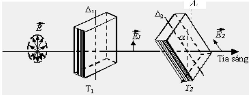
Hình 5-5a . Sơ đồ biểu diễn định luật Malus
