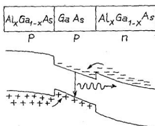
Hình 10.18. Sơ đồ chuyển tiếp dị thể GaAs – Al x Ga 1-x As
