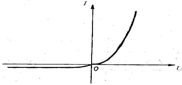
Hình 10-15. Đặc trưng Vôn – Ampe của diode.
