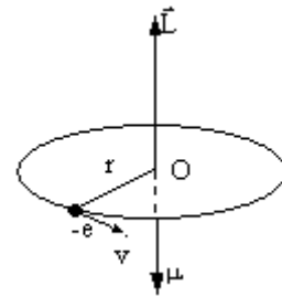
Hình 9-8. Mô hình nguyên tử cổ điển
