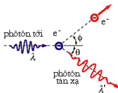
Hình 7-8. Va chạm đàn hồi giữa photon và electron
