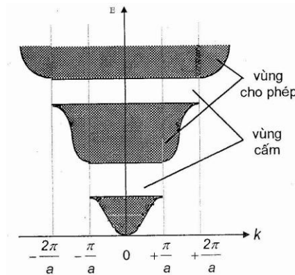
Hình 10-4: Sự phụ thuộc năng lượng của electron trong tinh thể vào số sóng k
