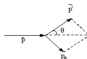
Hình 7-8. Bảo toàn động lượng
