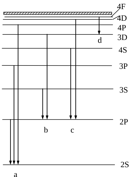
Hình 9-6. Sơ đồ quang phổ của Li
