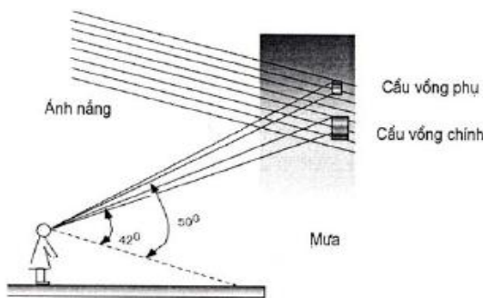
Hình 4-11. Góc quan sát cầu vòng
