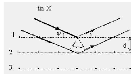
Hình 3-15. Nhiễu xạ trên tinh thể
