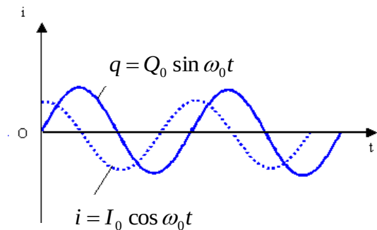
Hình 1-8. Đường biểu diễn dao động điều hoà
