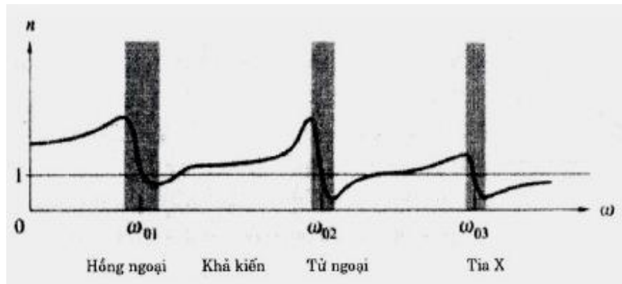
Hình 4-2. Sự tán sắc dị thường
