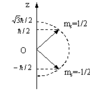
Hình 9-11. Sự lượng tử hóa không gian của spin
