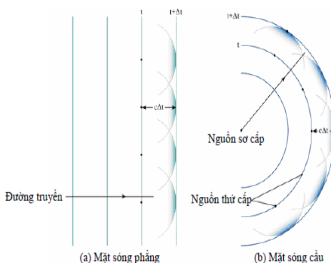
Hình 2-4. Mô tả nguyên lý Huygens
