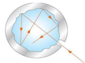
Hình 7-2. Vật đen tuyệt đối
