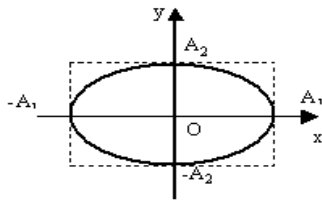
Hình 1-18. Quỹ đạo của chất điểm khi
