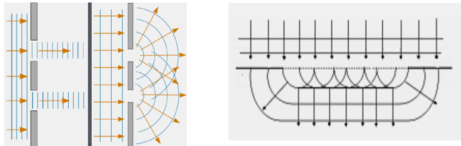
Hình 3-2. Giải thích định tính hiện tượng nhiễu xạ
