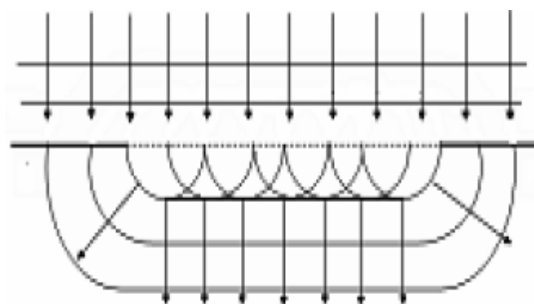
Hình 1-31: Hiện tượng nhiễu xạ sóng
