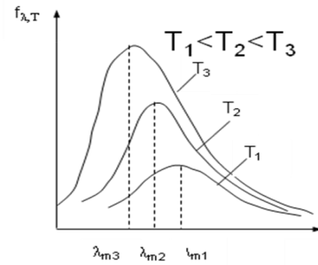
Hình 7-4b. Phổ phát xạ của vật đen tuyệt đối ở các nhiệt độ T_1 < T_2 < T_3
