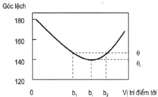
Hình 4-10. Góc lệch của tia sáng theo vị trí điểm tới giọt mưa.
