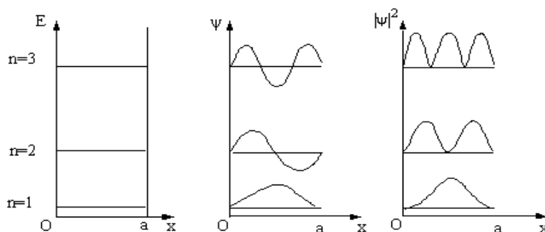
Hình 8-7. Vật thể vi mô trong giếng thế năng một chiều, cao vô hạn
