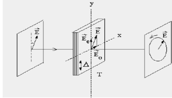
Hình 5-11. Ánh sáng phân cực elip
