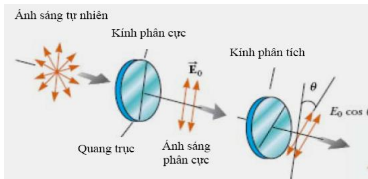
Hình 5-5b. Phương pháp phân cực ánh sáng bằng kính phân cực
