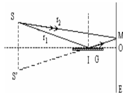
Hình 2-12. Thí nghiệm của Lloyd
