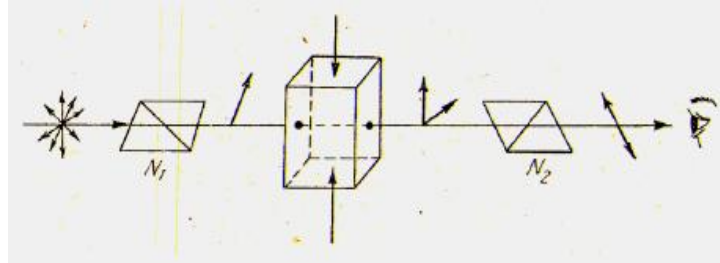
Hình 5-15. Sơ đồ nghiên cứu hiện tượng lưỡng chiết do biến dạng.
