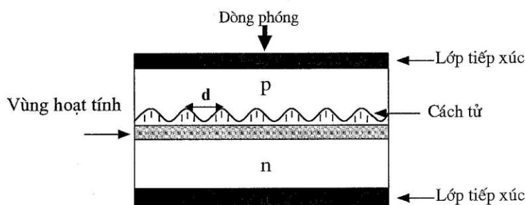
Hình 10.19. Cấu trúc điốt laser phản hồi phân tán.
