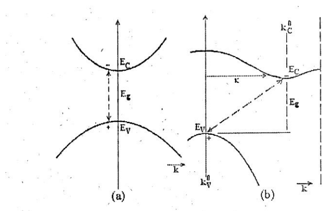
Hình 10-5: Sơ đồ vùng năng lượng của bán dẫn vùng cấm thẳng (a) và bán dẫn vùng cấm xiên (b)
